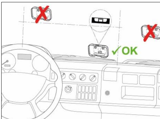
Imagine 8: Amplasarea corectă a OBU pe parbriz
