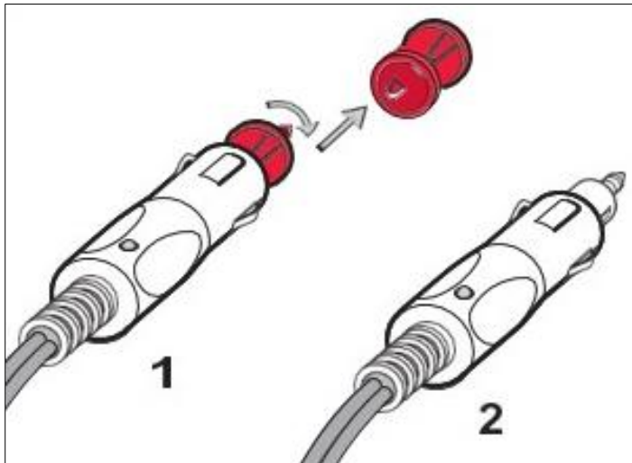
Imagine 12: Racord electric la montajul flexibil
